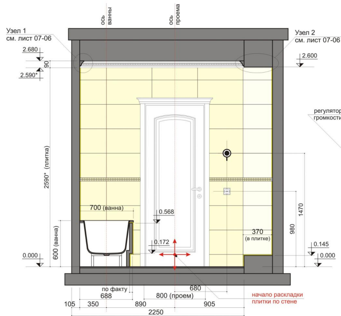
Вид В
