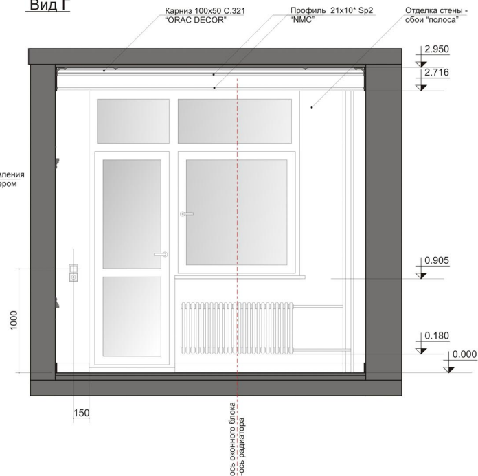
Вид Г
