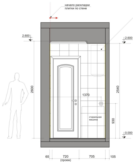
Вид А
