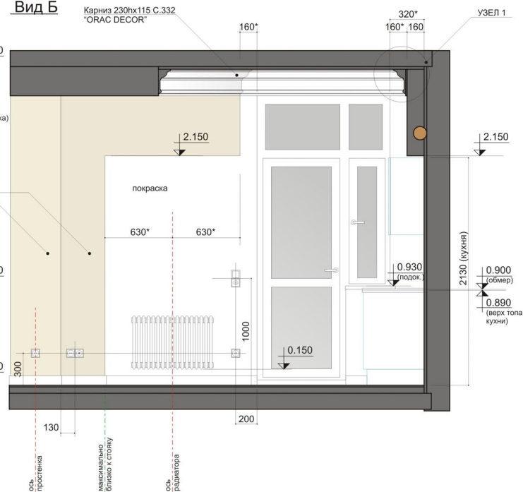
Вид Б
