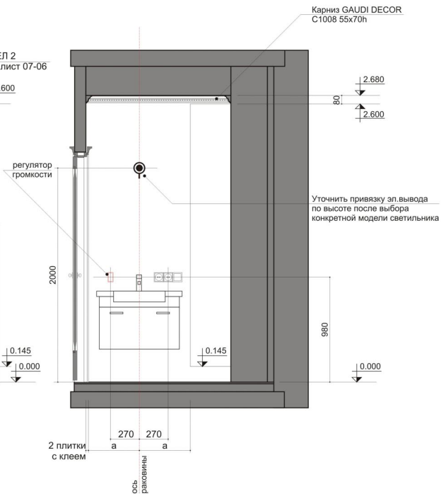
Вид Г
