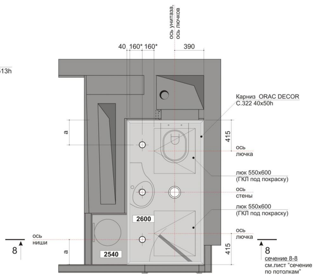
План потолка
