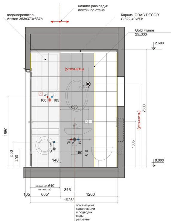
Вид Б
