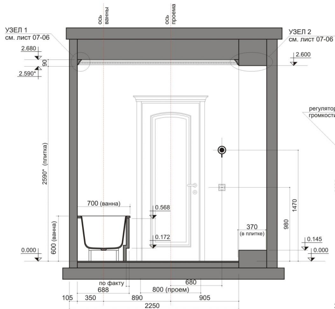
Вид В
