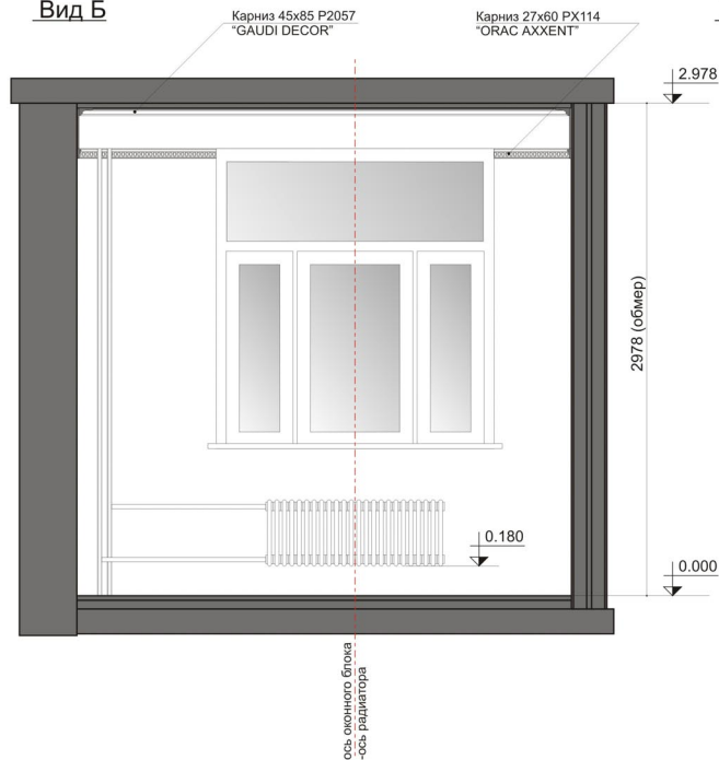
Вид Б
