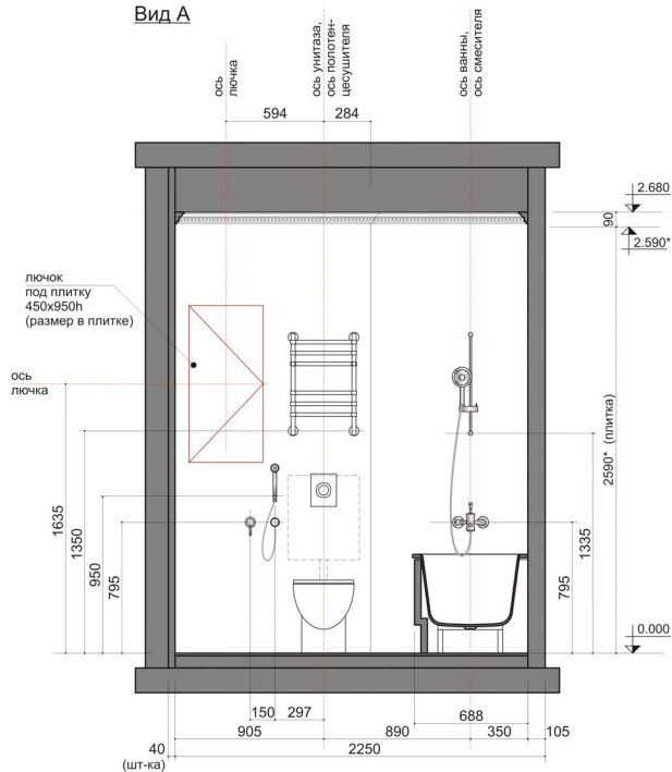
Вид А
