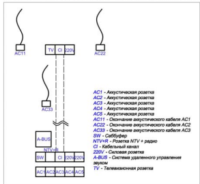
СХЕМА РОЗЕТОК ДЛЯ ДОМАШНЕГО КИНОТЕАТРА
