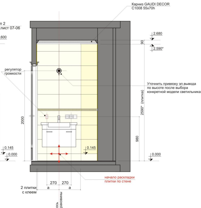
Вид Г
