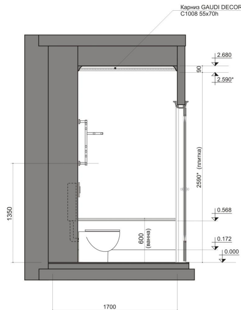
Вид Б
