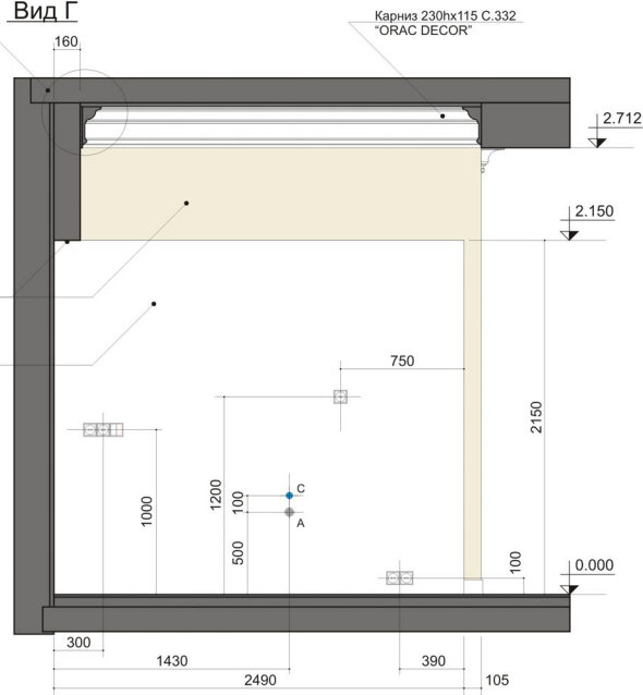
Вид Г
