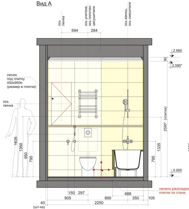
Вид А
