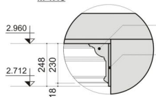
УЗЕЛ 1 М 1:15
