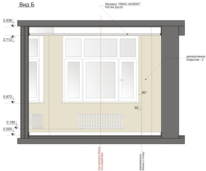
Вид Б
