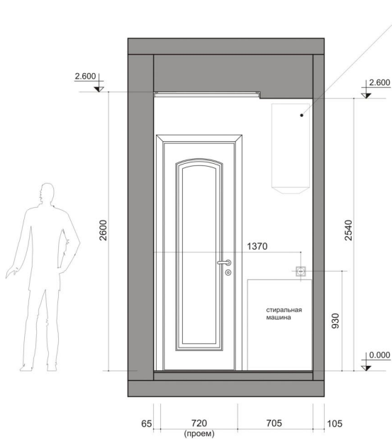
Вид А
