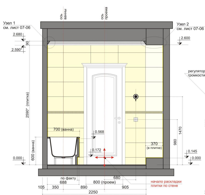
Вид В
