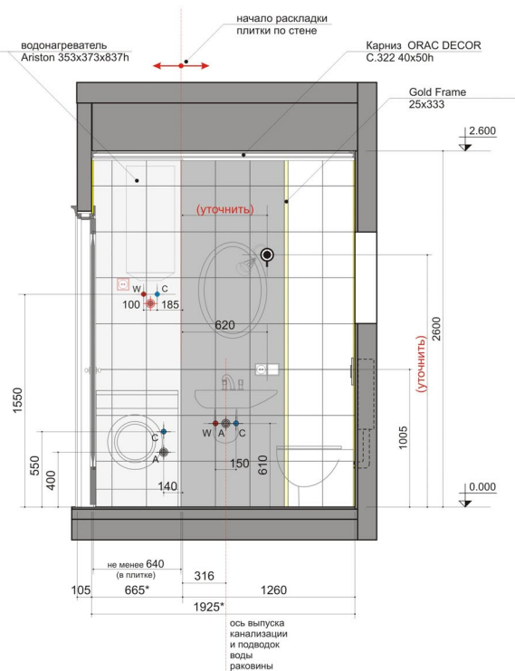
Вид Б
