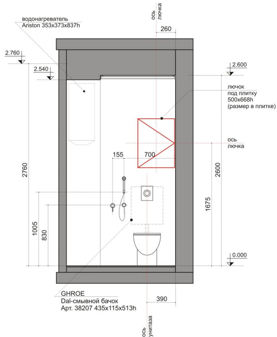
Вид В
