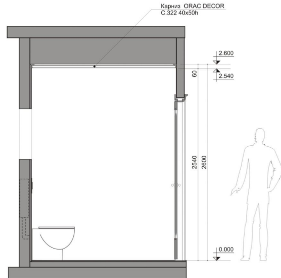
Вид Г
