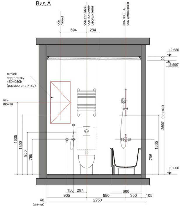
Вид А
