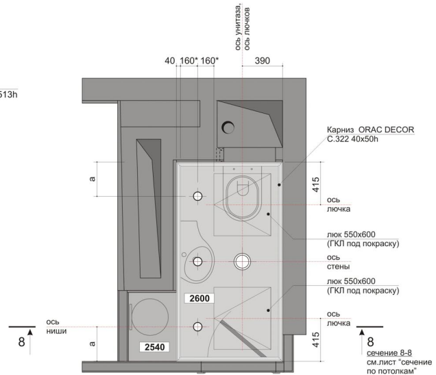
План потолка
