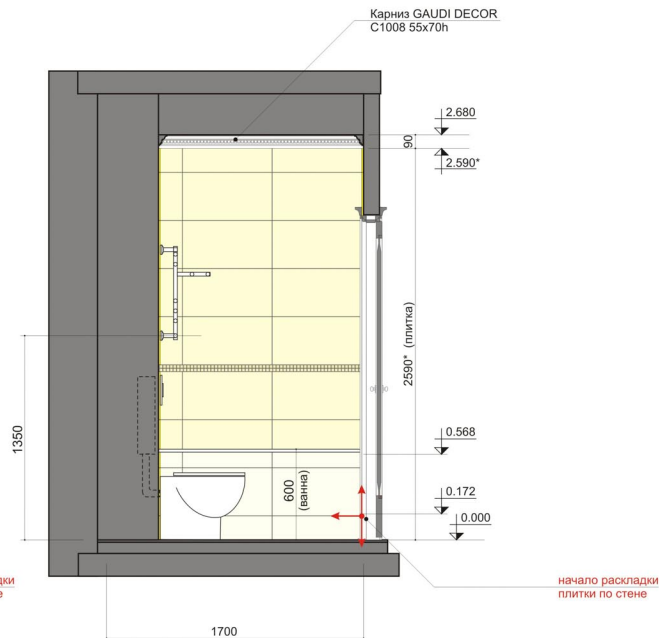
Вид Б
