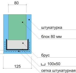
Узел 2 М 1:5
