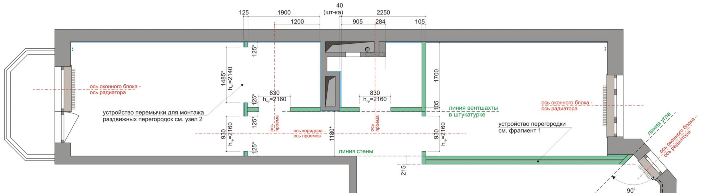
Фрагмент 1 М 1:15
