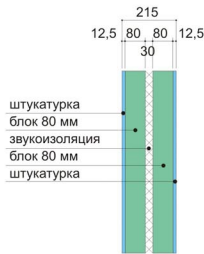
Фрагмент 1 М 1:15
