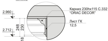
УЗЕЛ 1 М 1:15
